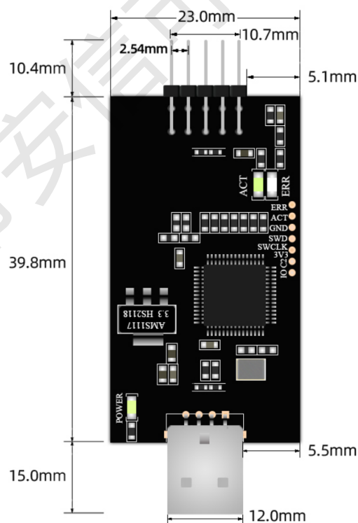
图 3 开发板尺寸图
