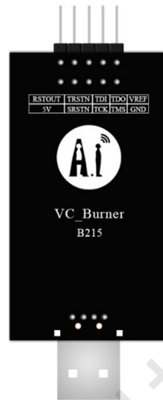
图 5 调试器管脚示意图（底部视图）
