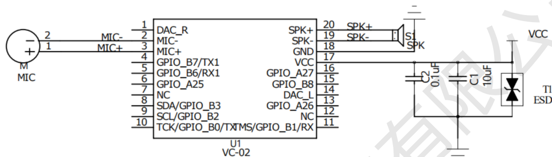
图 7 应用电路图
