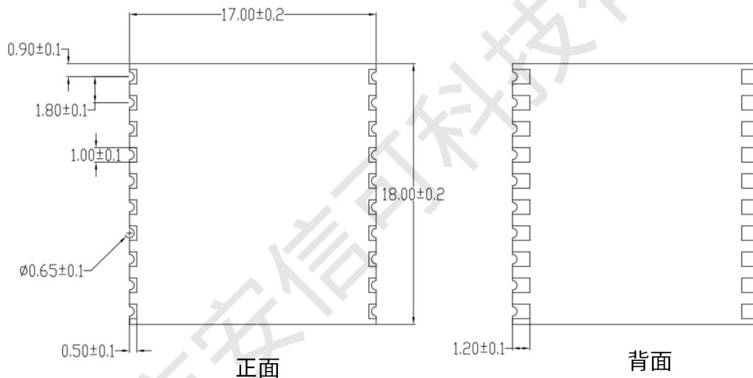
图 4 模组尺寸图
