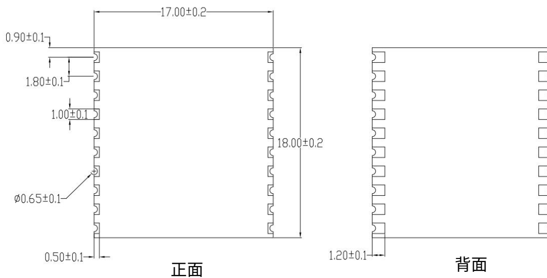
图 4 模组尺寸图
