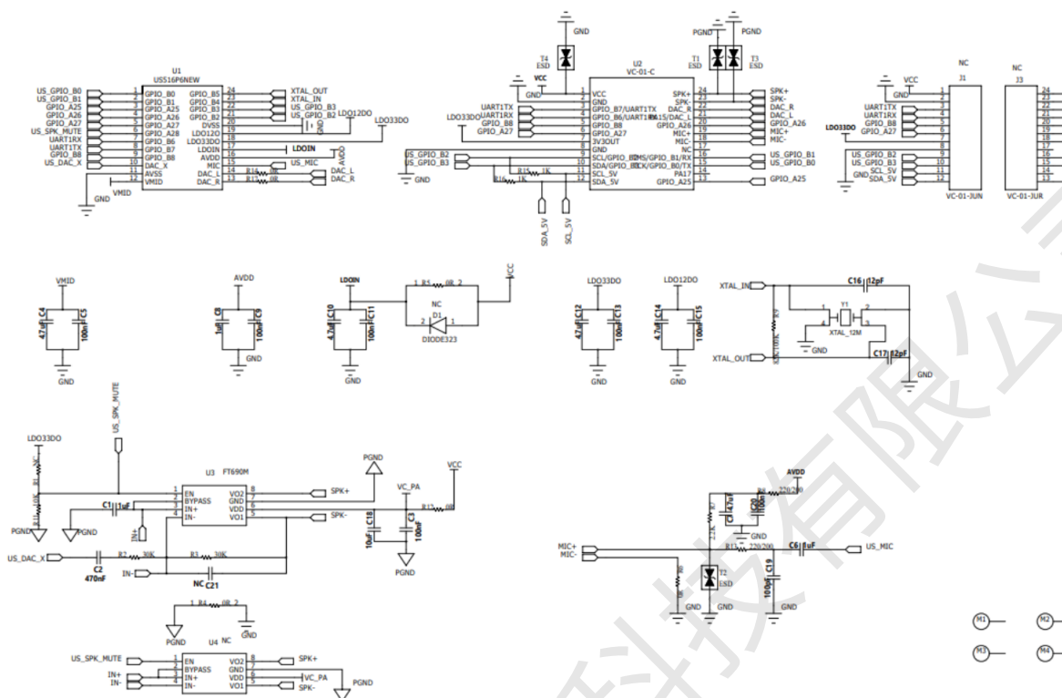
图 6 模組原理图
