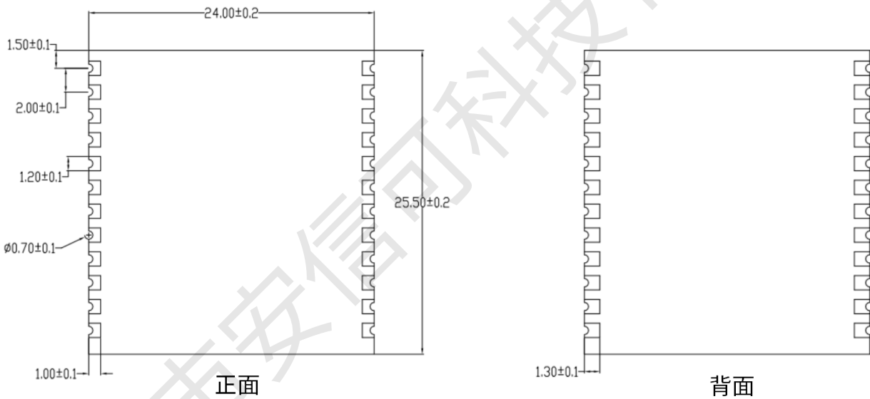
图 4 模组尺寸图
