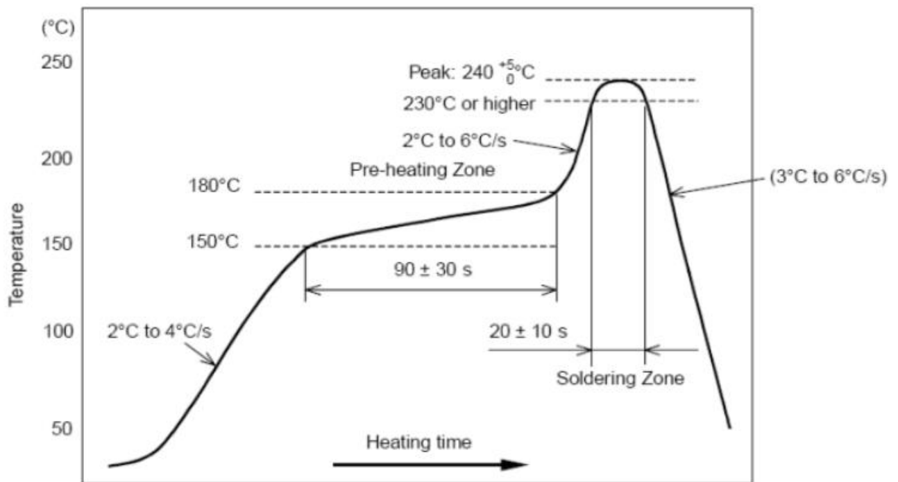
图 12 回流焊曲线图
