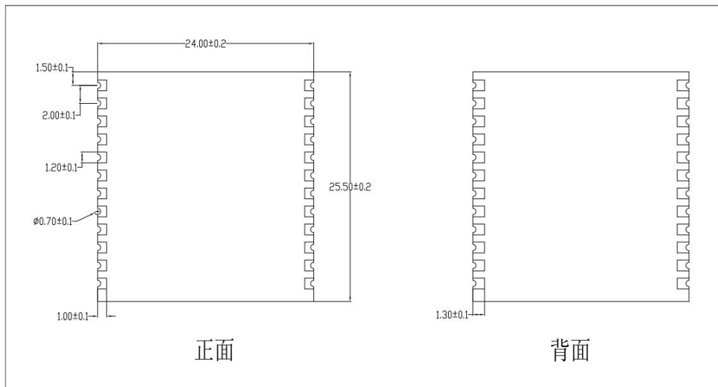
图 4VB-01 尺寸图
