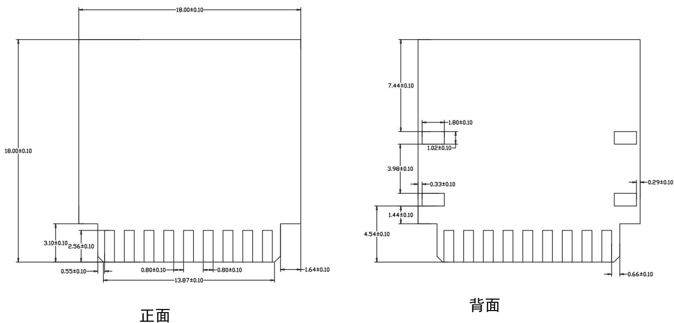
图 4 模組尺寸图
