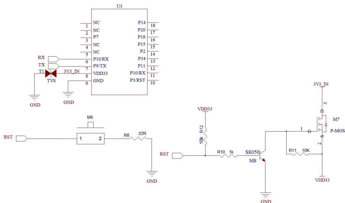
图 10 应用电路图
