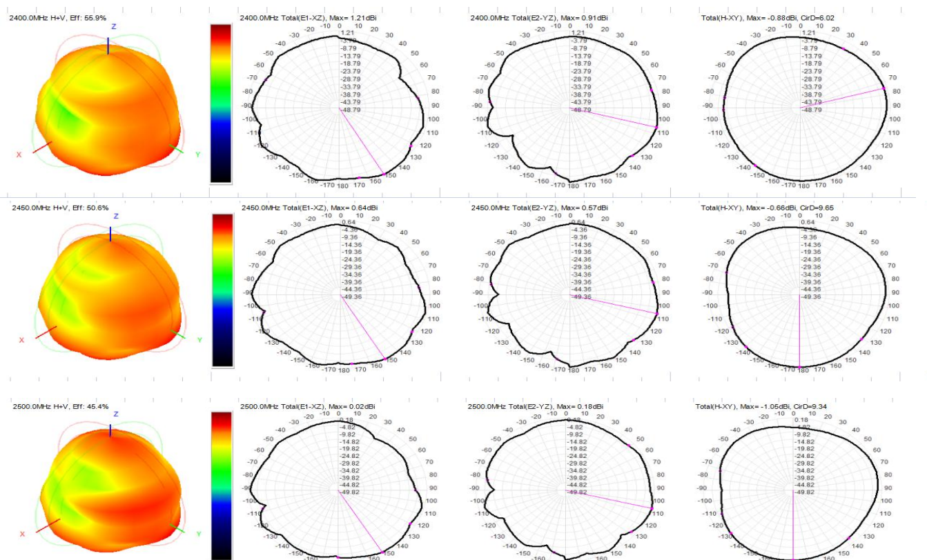
图 9 天线场型图
