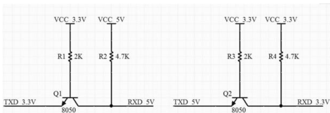
图 13 电平转换电路
