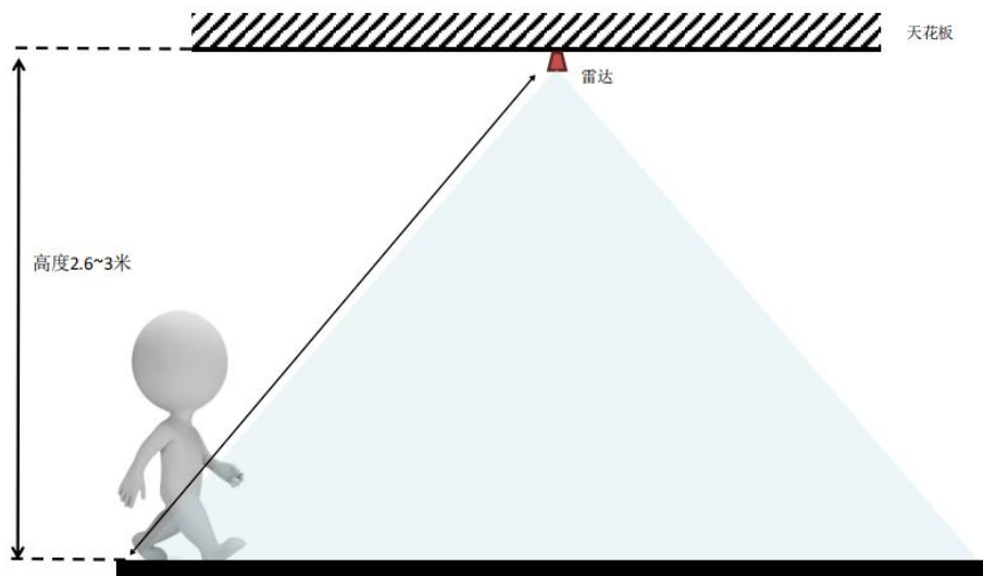
图 8 挂顶安装示意图
