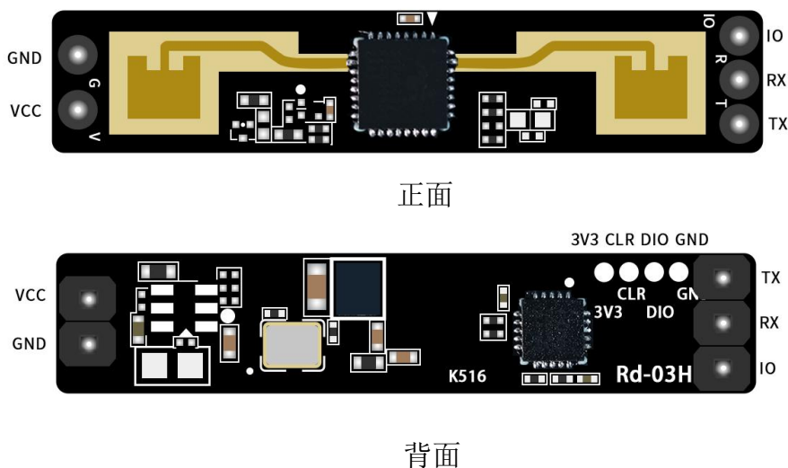
图 5 管脚示意图
