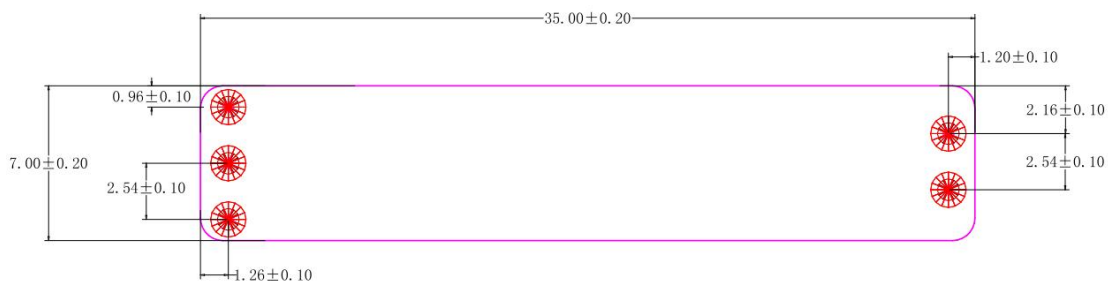
图 4 尺寸图（单位：mm）
