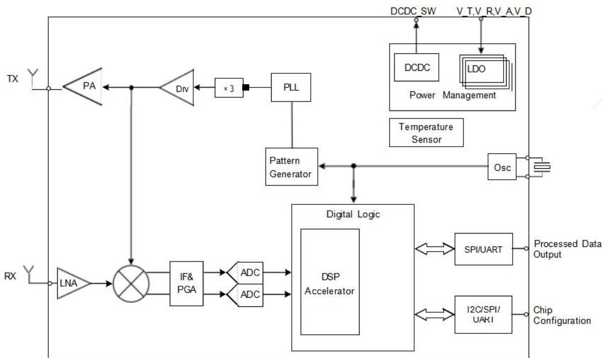
图 1 S1KM0000 芯片架构图
