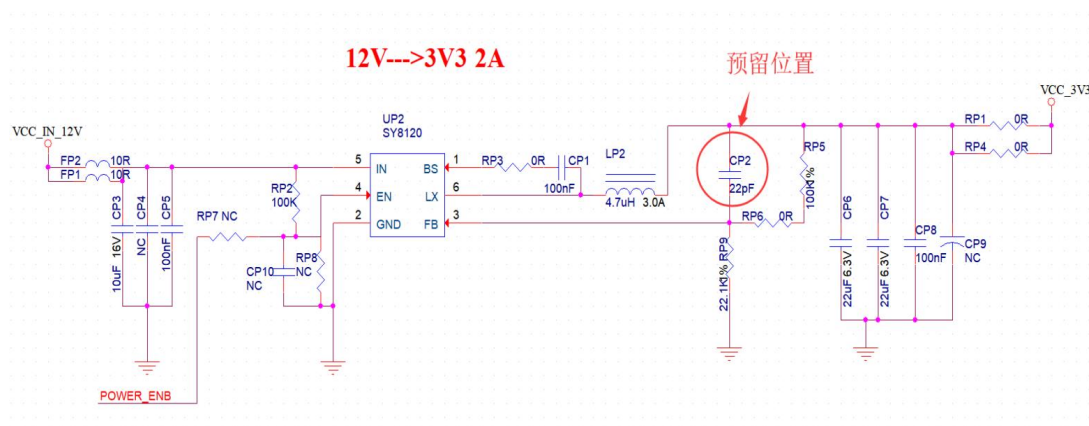
图 12 DC-DC 降压电路图
