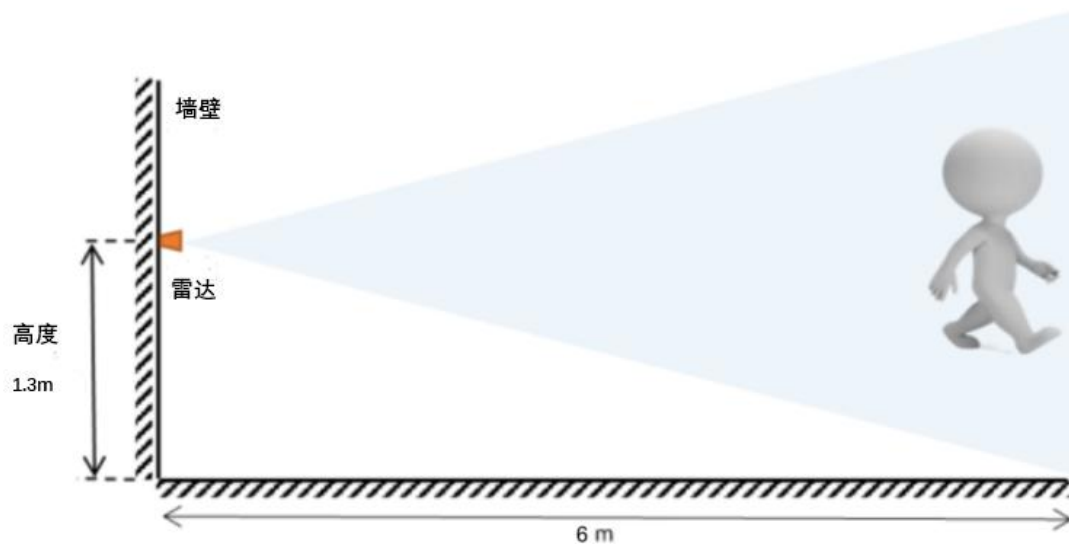
图 9 精准测距挂壁安装示意图
