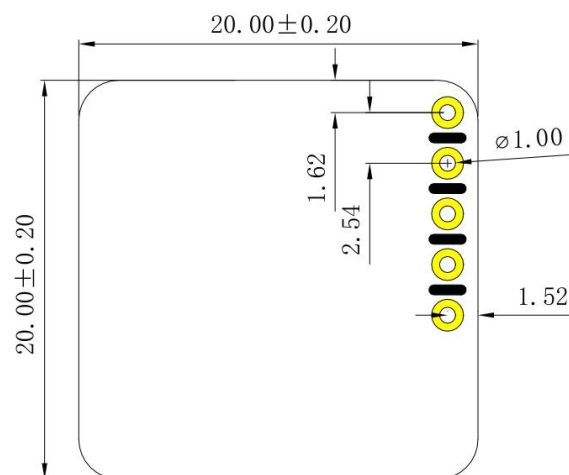
图 8 推荐 PCB 封装尺寸
