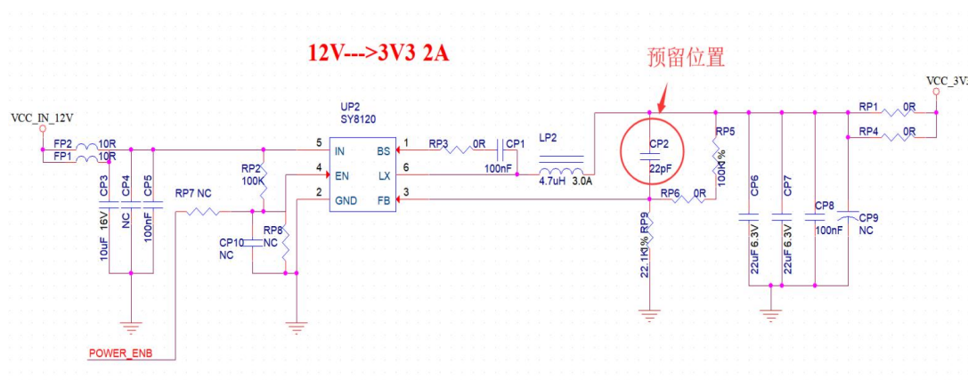
图 15 DC-DC 降压电路图
