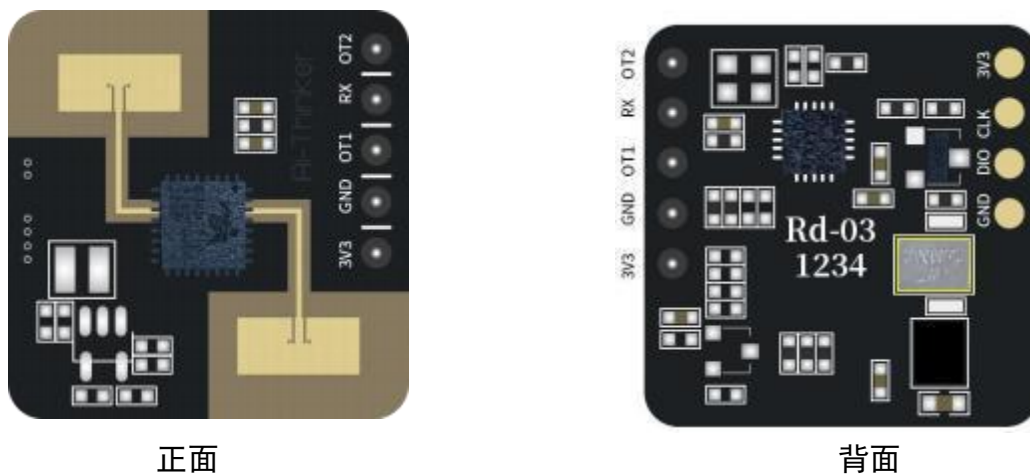
图 1 管脚示意图
