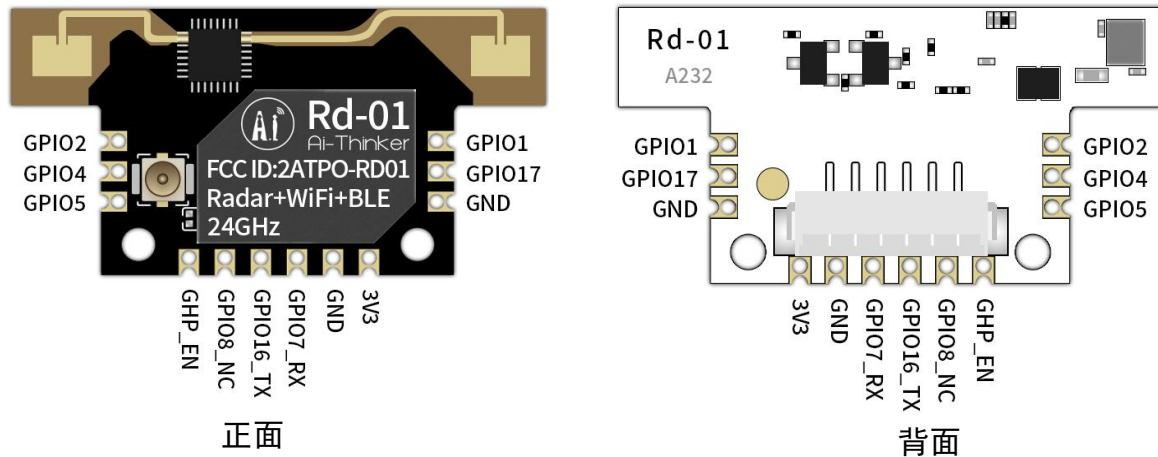
图 6 管脚示意图
