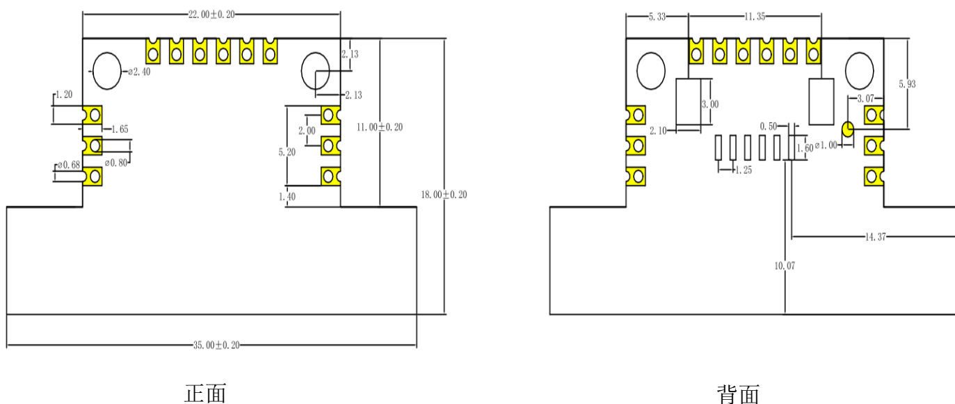
图 5 尺寸图
