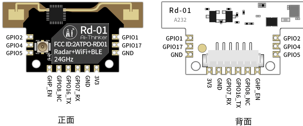
图 6 管脚示意图
