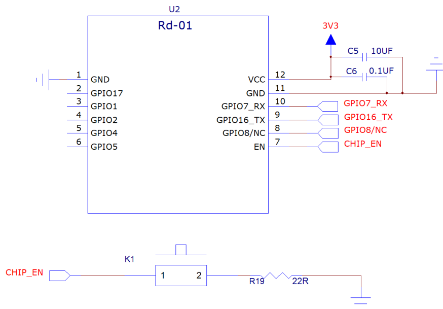
图 8 应用指导电路
