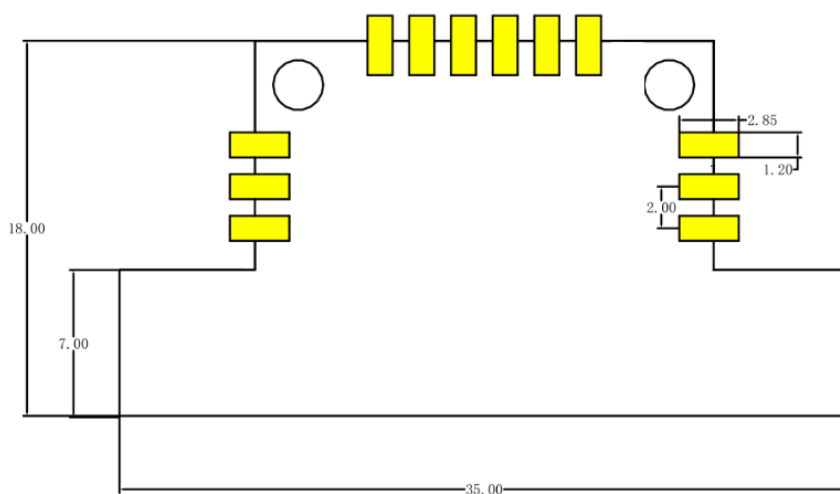
图 9 推荐 PCB 封装尺寸
