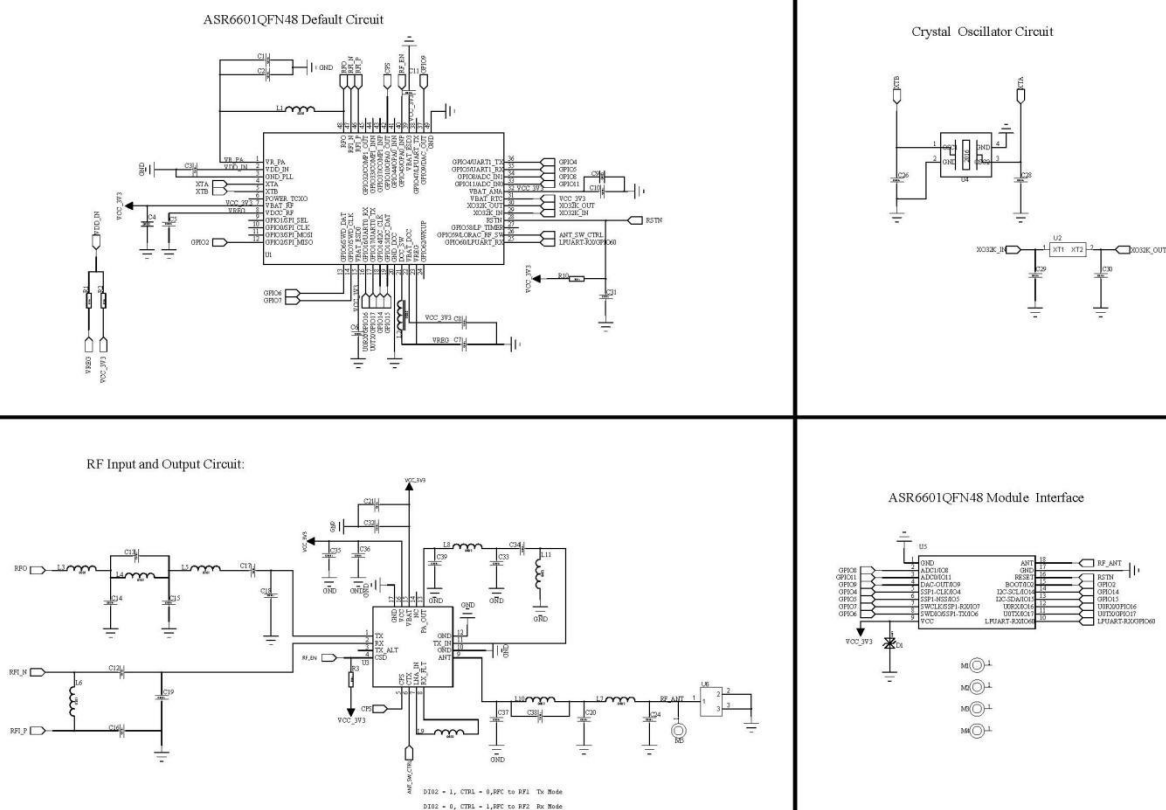
图 6 原理图
