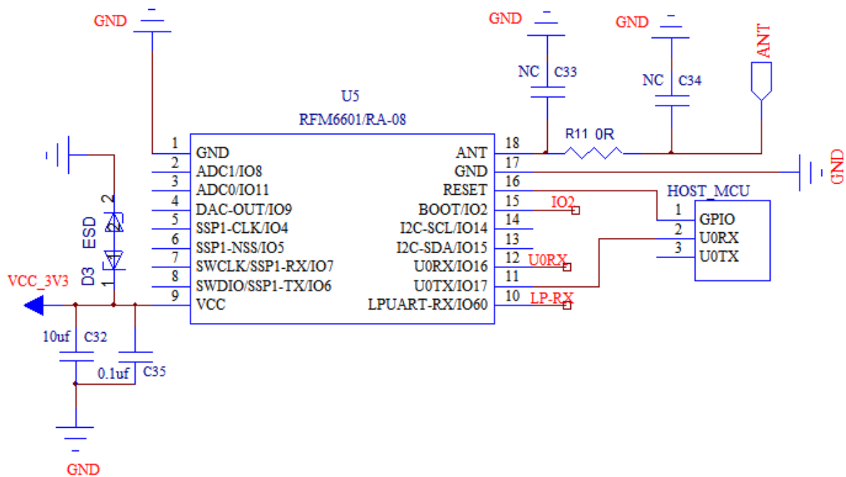
图 7 应用电路图
