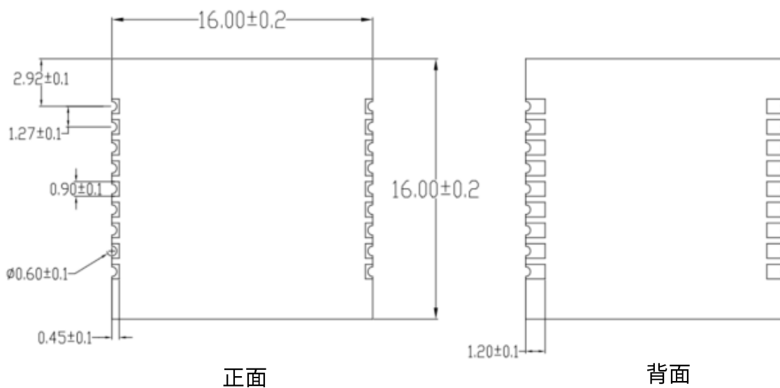
图 4 模组尺寸图
