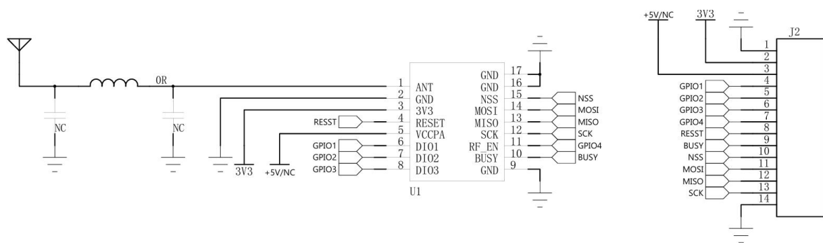
图 7 典型应用电路
