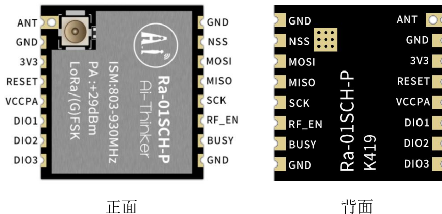
图 5 管脚示意图
