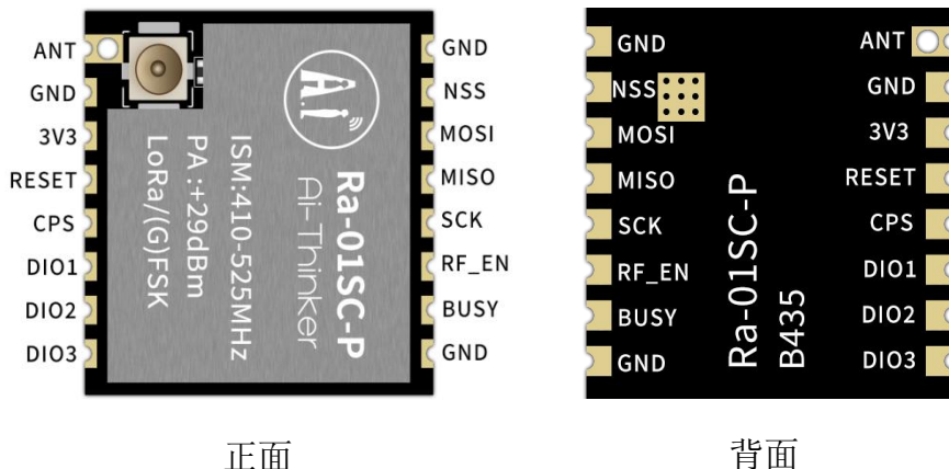
图 5 管脚示意图
