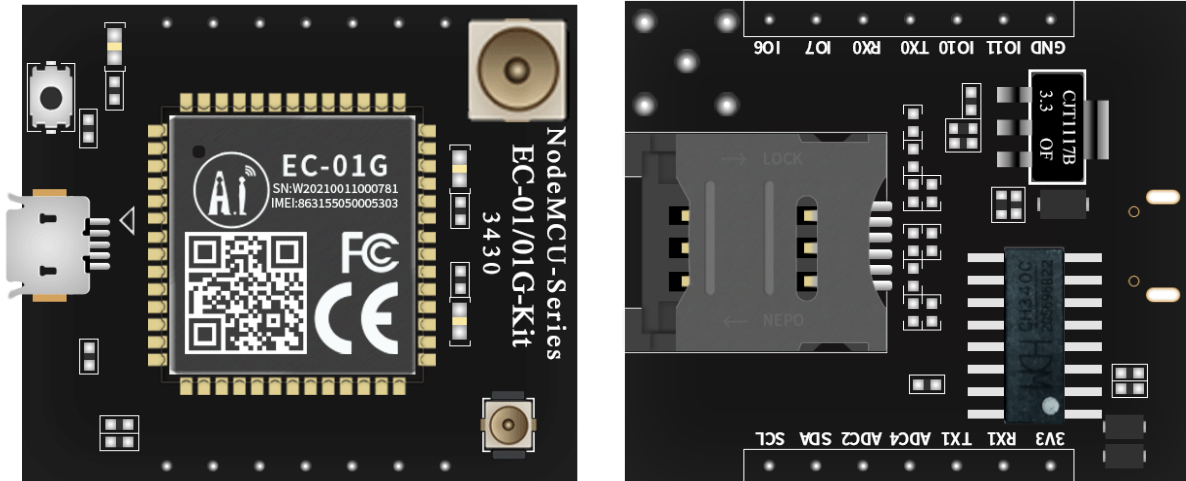
图 2 开发板外观图(图片及丝印仅供参考，以实物为准)
