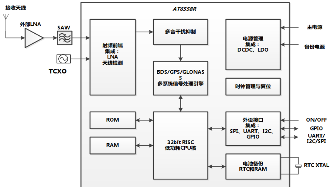
图 1 AT6558R 芯片架构图
