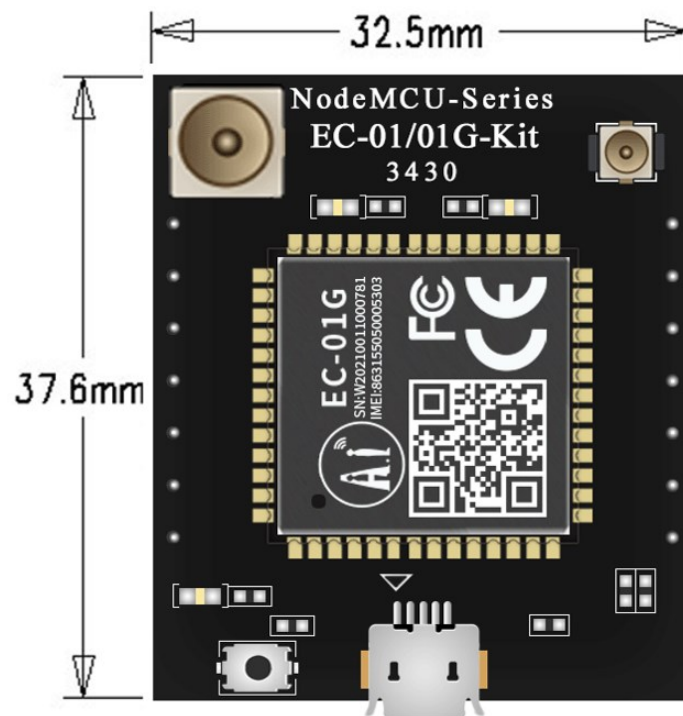
图 5 开发板尺寸图
