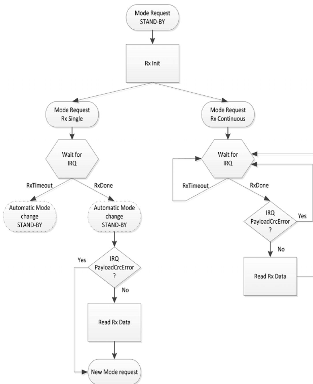
图 10 LoRa TM 接收序列
