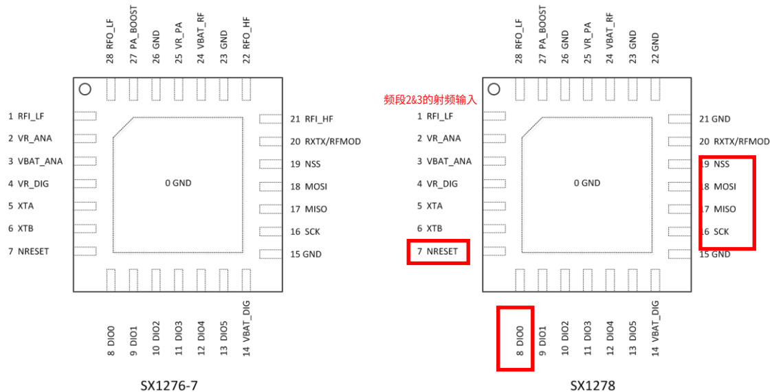
图 2 引脚图
