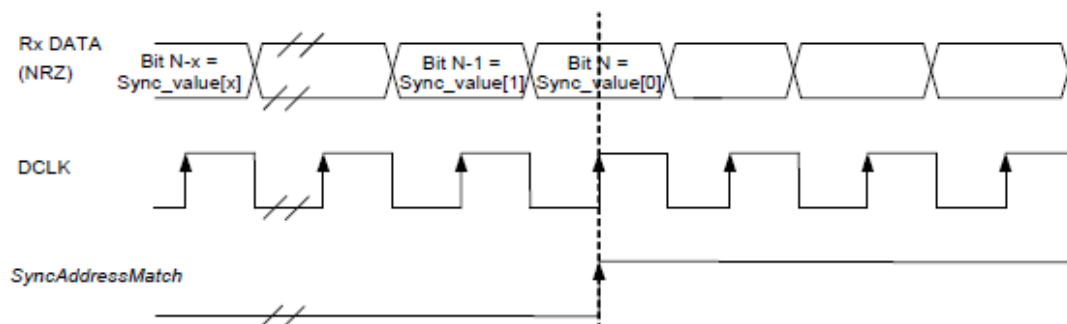
图 28 同步字识别
