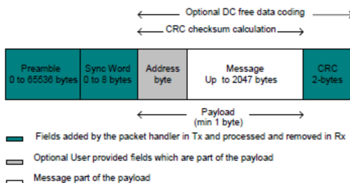
图 33 固定长度数据包格式
