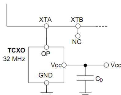
图 39 TCXO 连接
