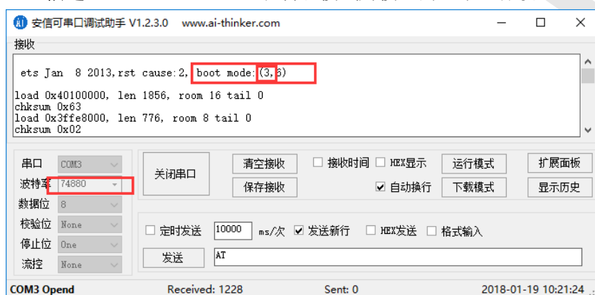
图 18: 正常模式
