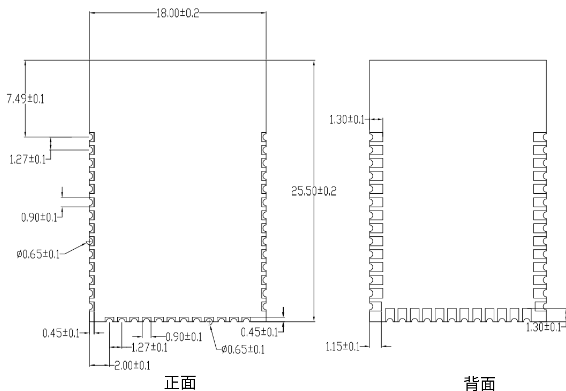
图 5 模组尺寸图
