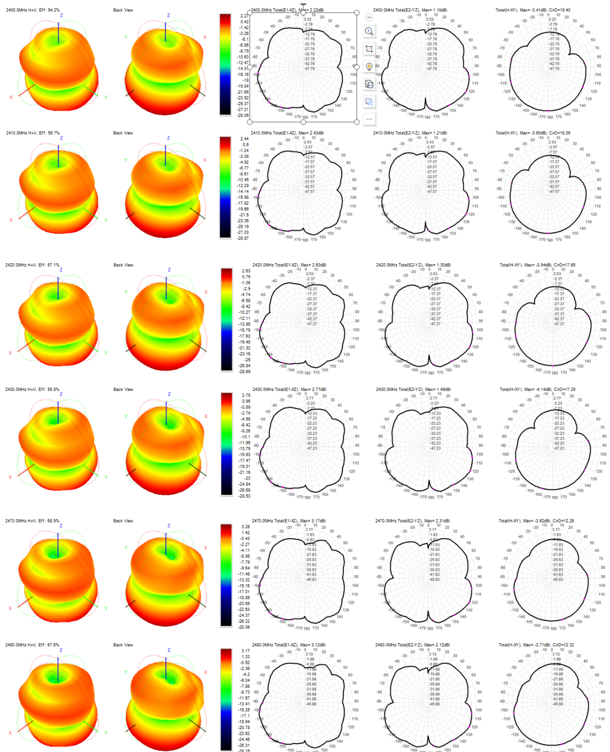
图 10 天线场型图
