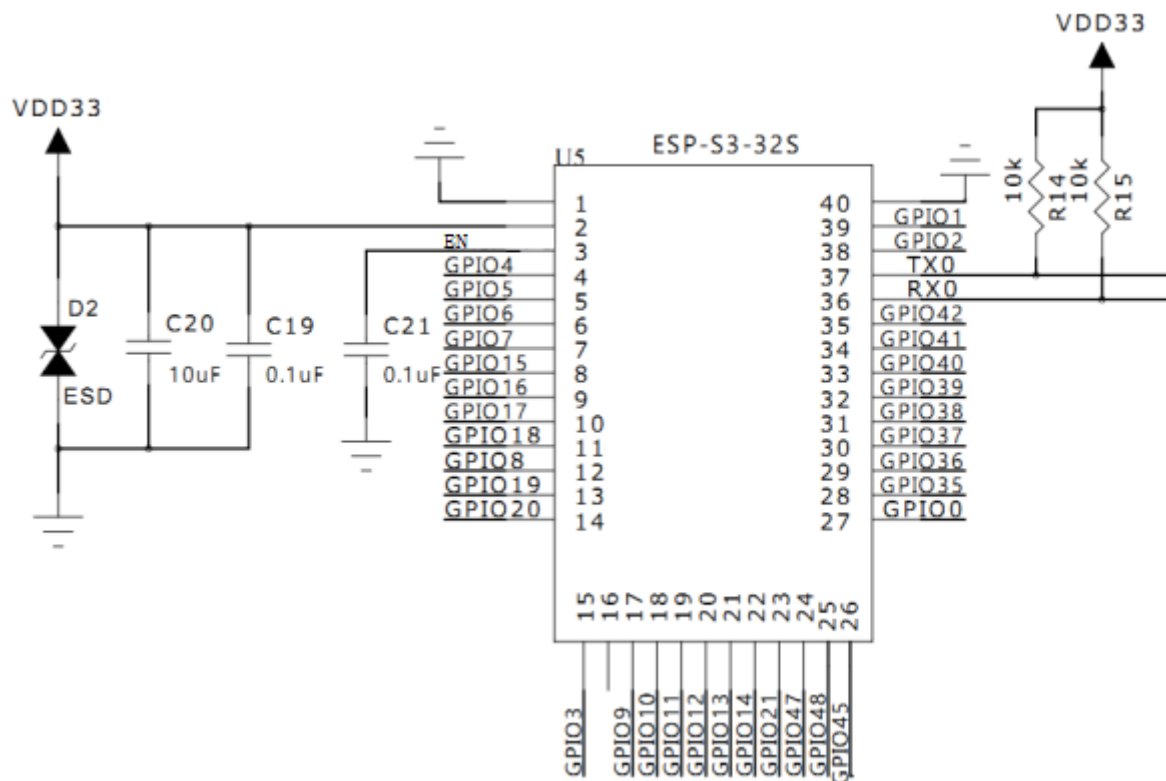
图 11 应用电路图
