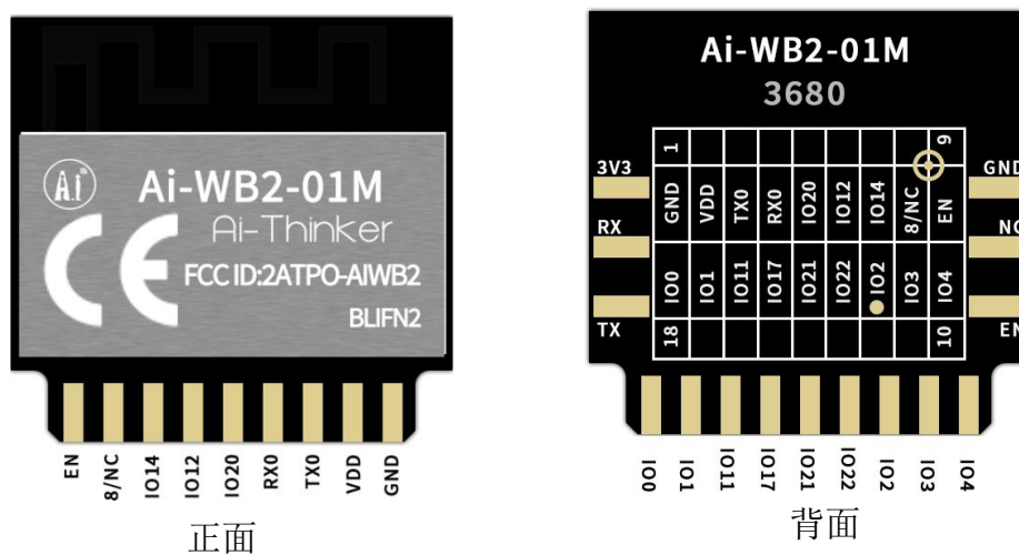
图 6 管脚示意图
