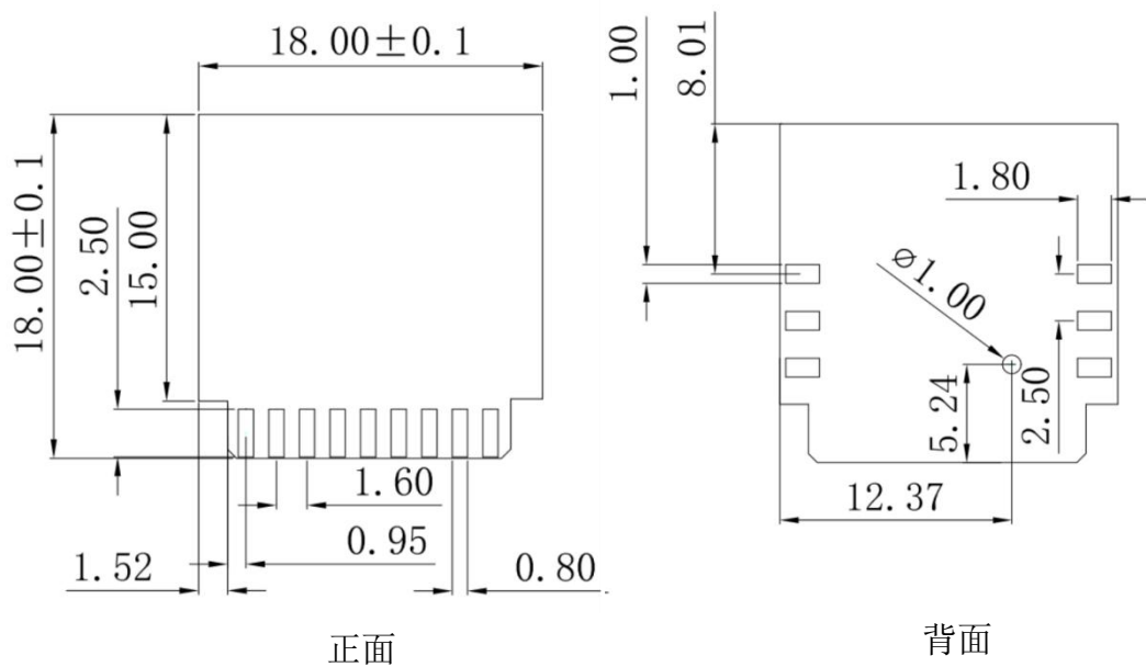
图 4 尺寸图
