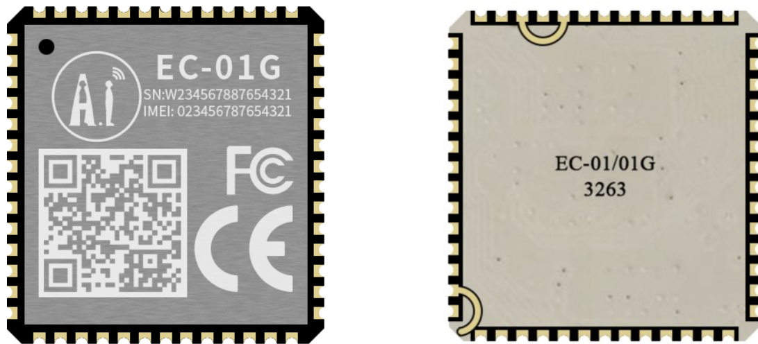
图 4 EC-01G 外观图(图片及丝印仅供参考，以实物为准)
