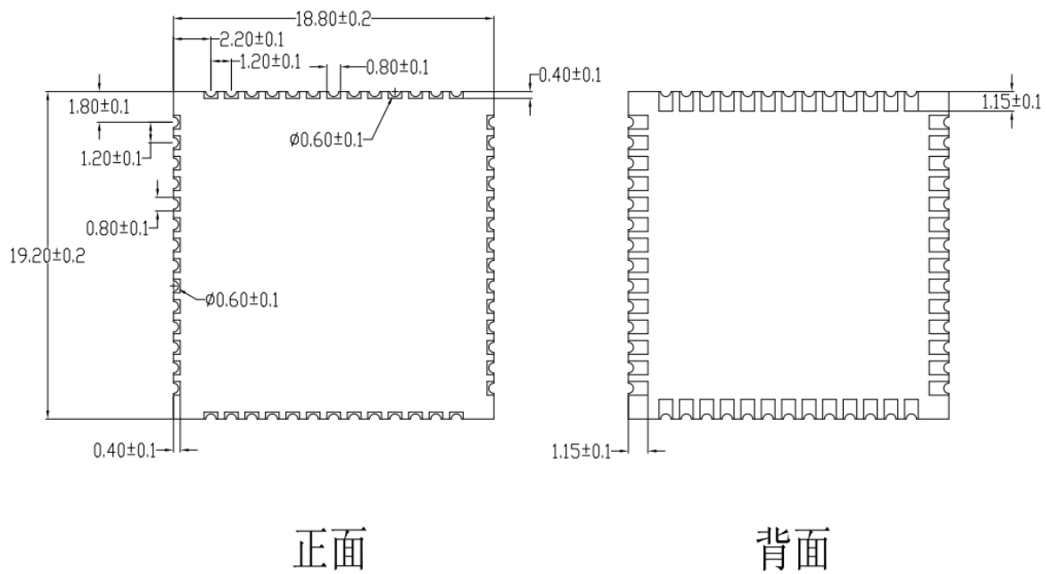
图 5 模组尺寸图
