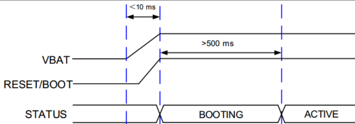
图 11 NB 芯片上电时序图
