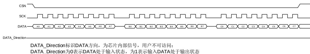
图 5-1 SPI 写操作
