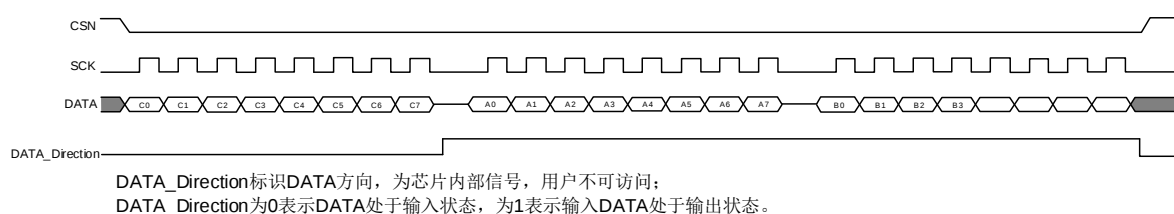
图 5-2 SPI 读操作
