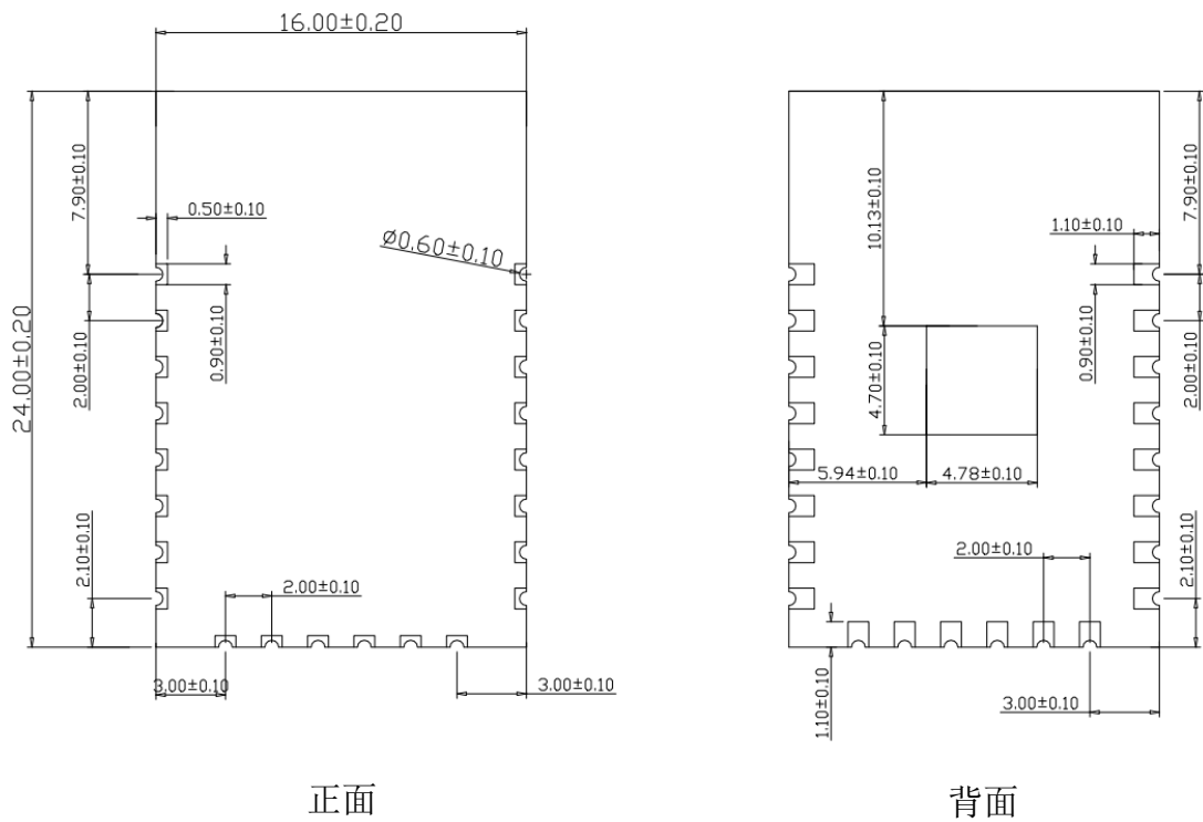
图 4 尺寸图
