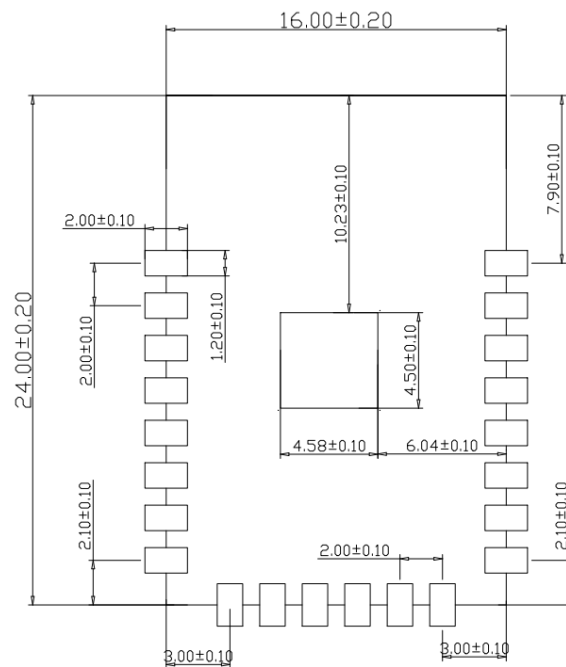
图 9 推荐 PCB 封装尺寸 (TOP 视图)
