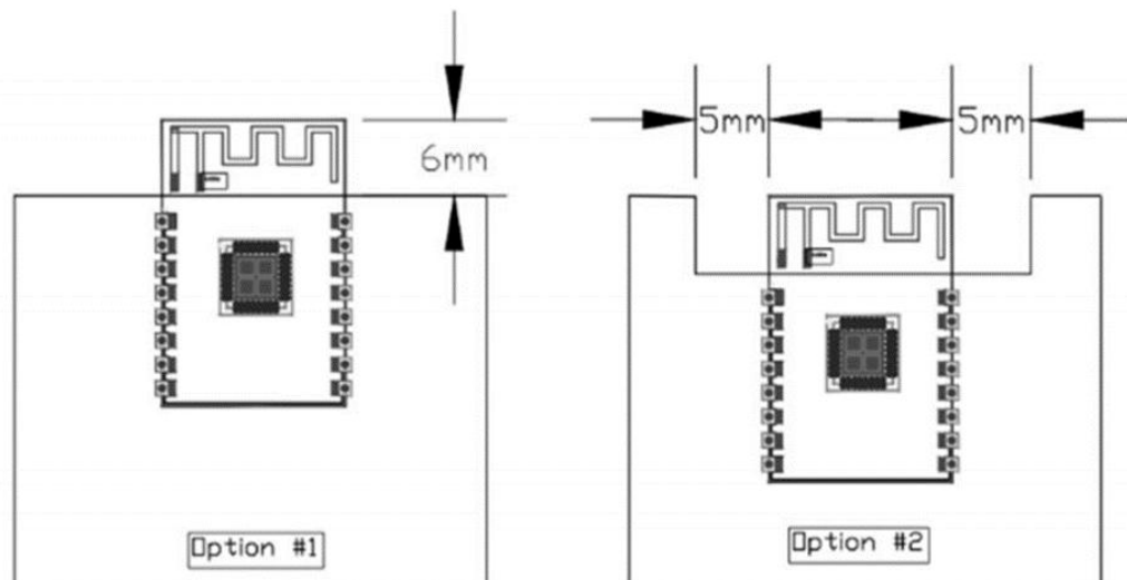
图 10 天线布局示意图
