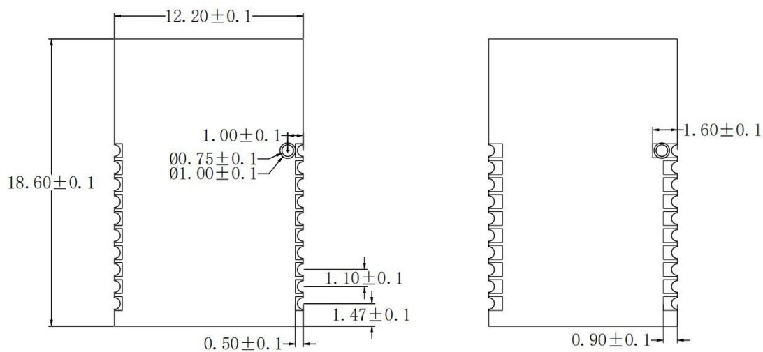
图 4 尺寸图（单位：mm）
