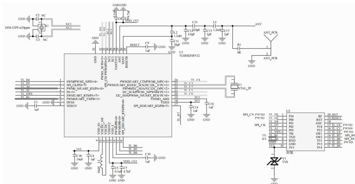
图 6 原理图
