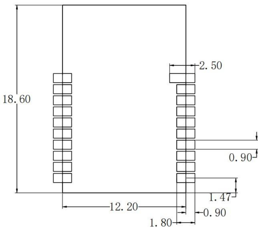
图 11 推荐 PCB 封装尺寸(单位: mm)
