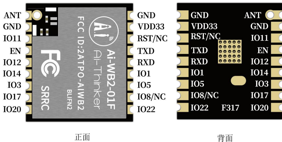
图 6 管脚示意图
