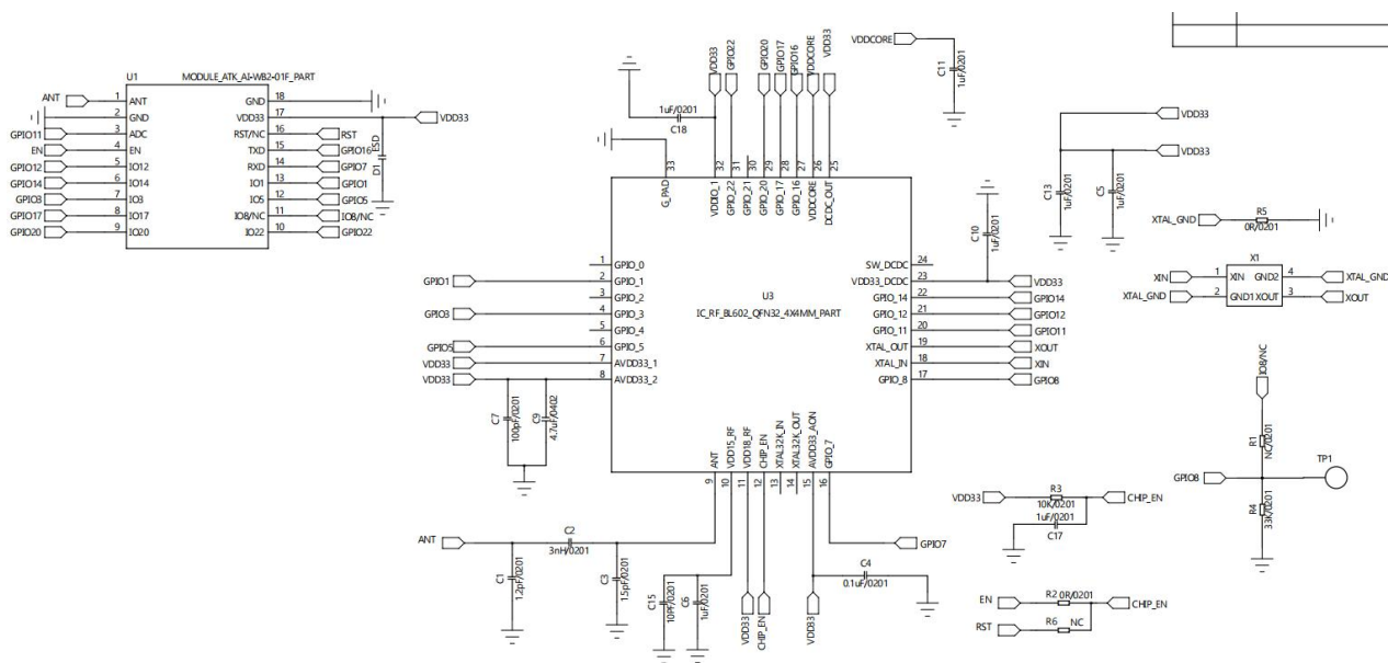
图 7 原理图
