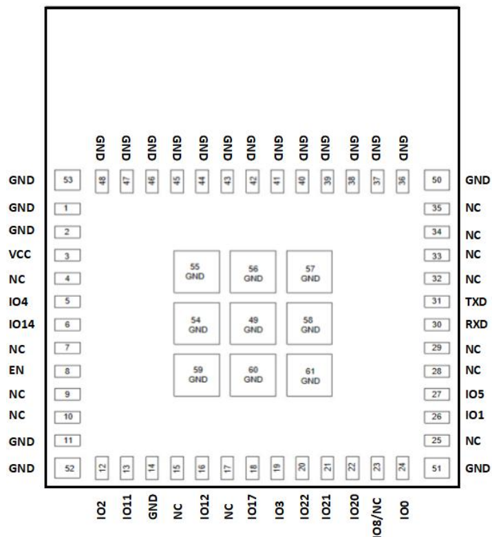
图 6 管脚顶视图
