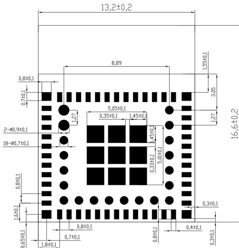
图 4 尺寸图
