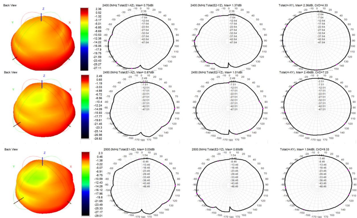
图 10 天线场型图
