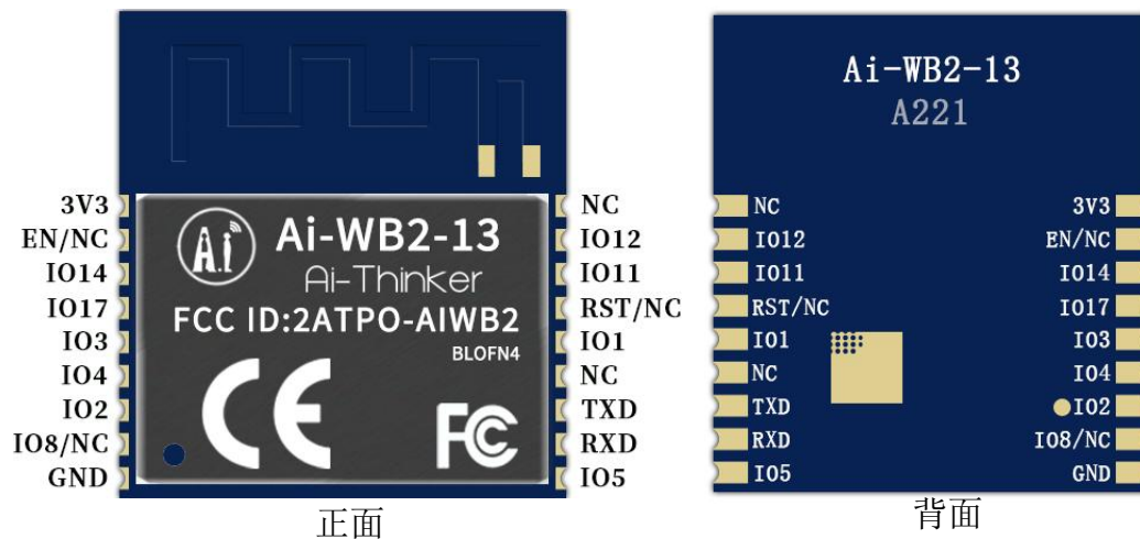
图 6 管脚示意图
