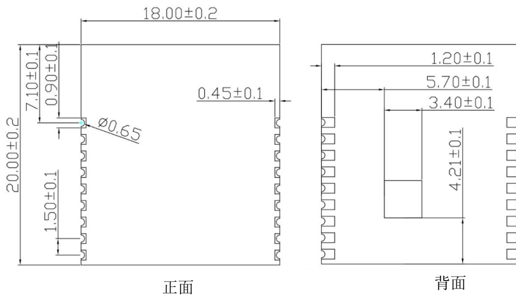
图 4 尺寸图
