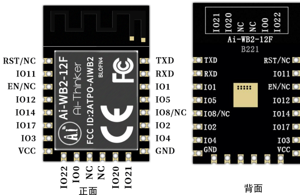
图 6 管脚示意图
