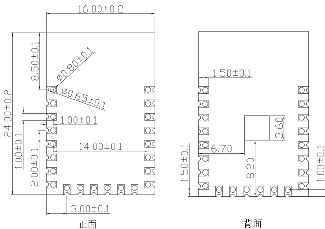
图 4 尺寸图
