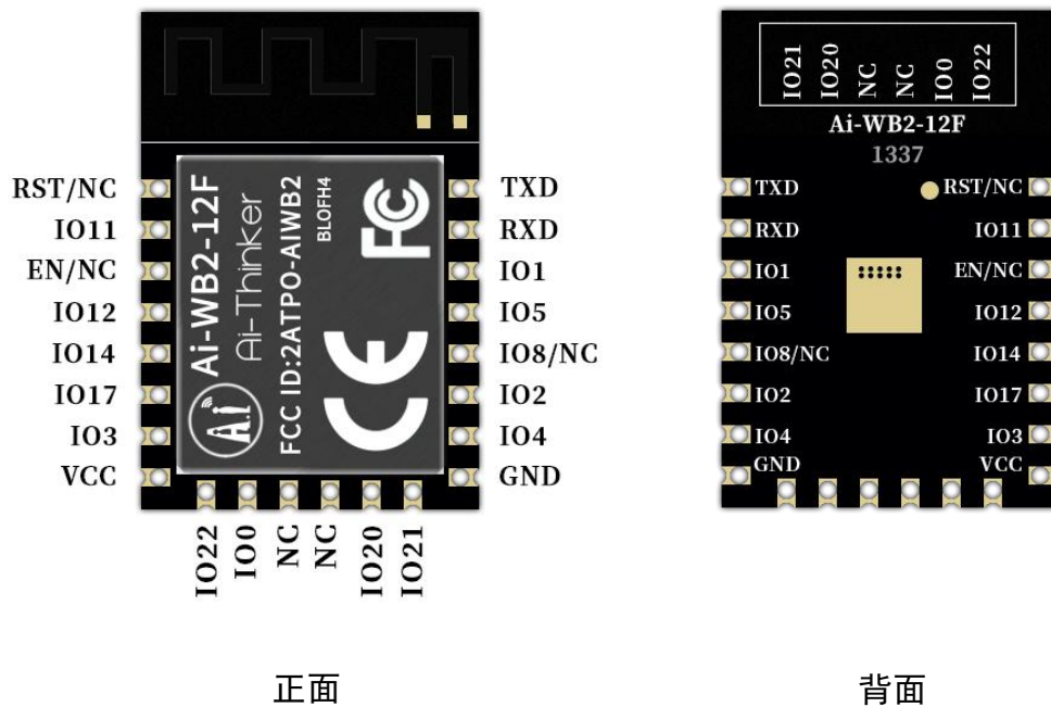
图 6 管脚示意图
