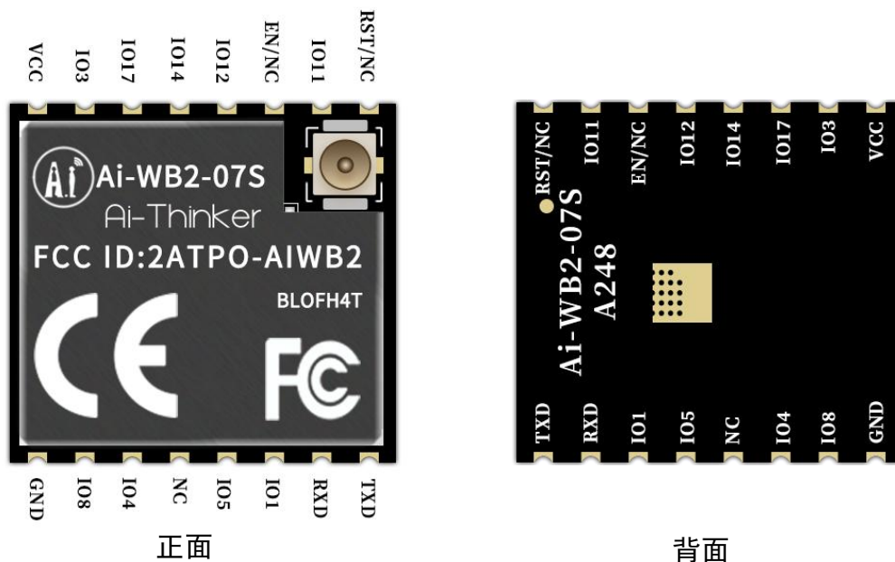
图 6 管脚示意图
