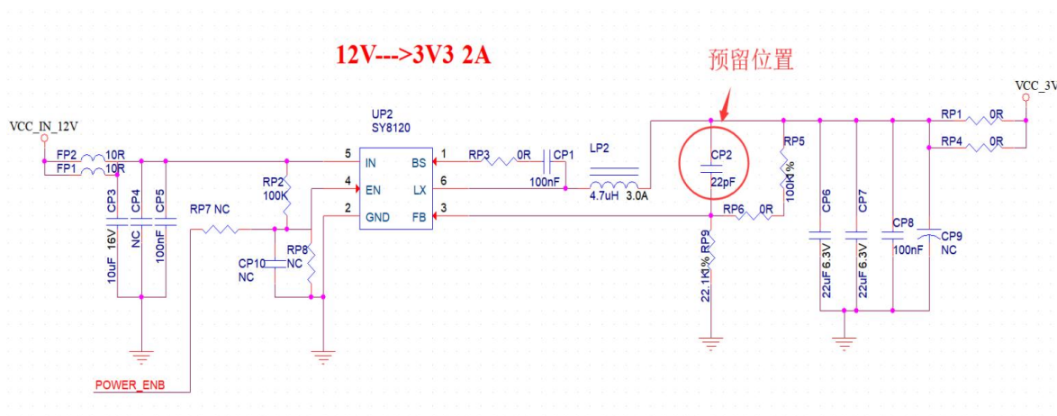
图 10 DC-DC 降压电路图
