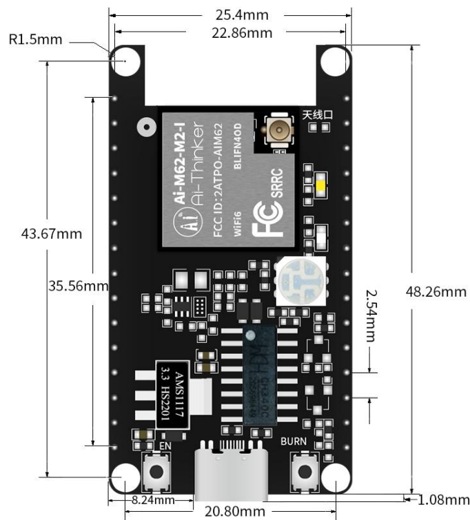
图 3 外观图（渲染图仅供参考，以实物为准）
