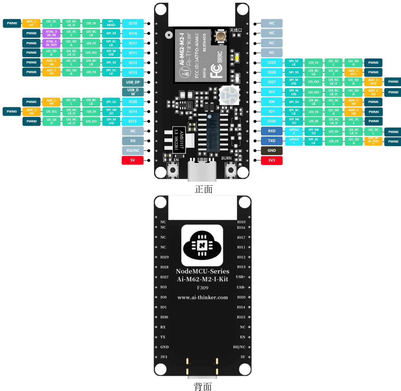
图 6 管脚示意图
