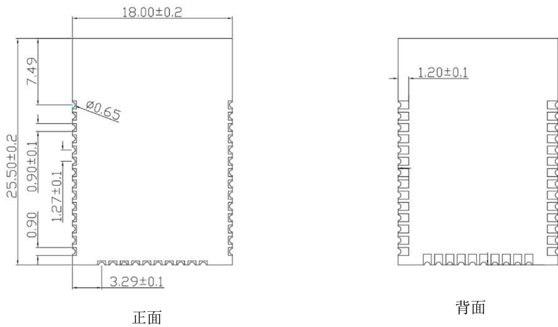
图 4 尺寸图
