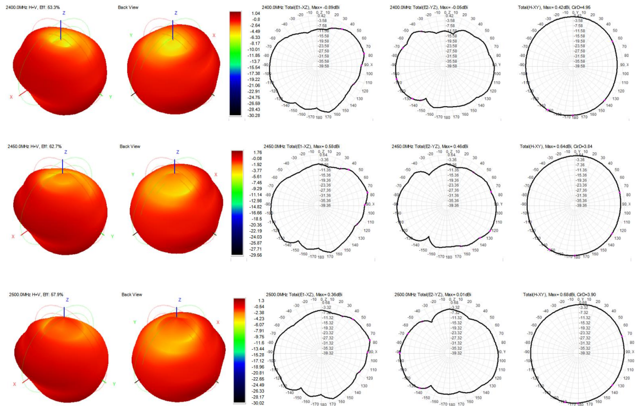
图 10 天线场型图
