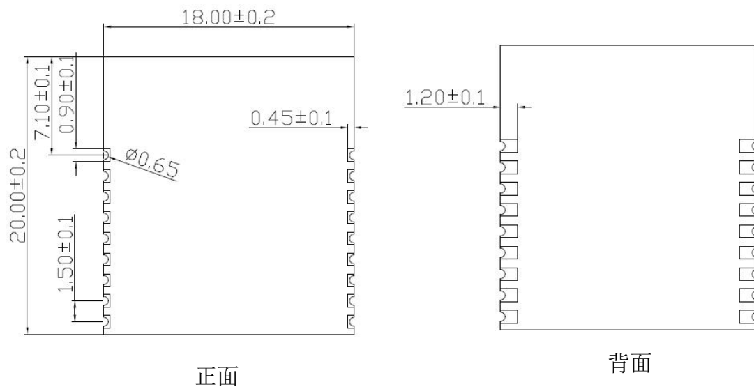
图 4 尺寸图
