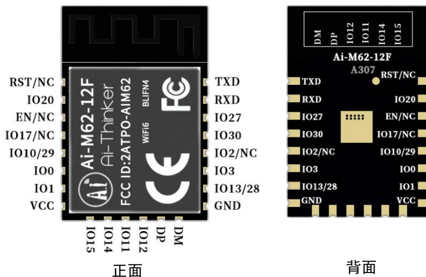
图 6 管脚示意图
