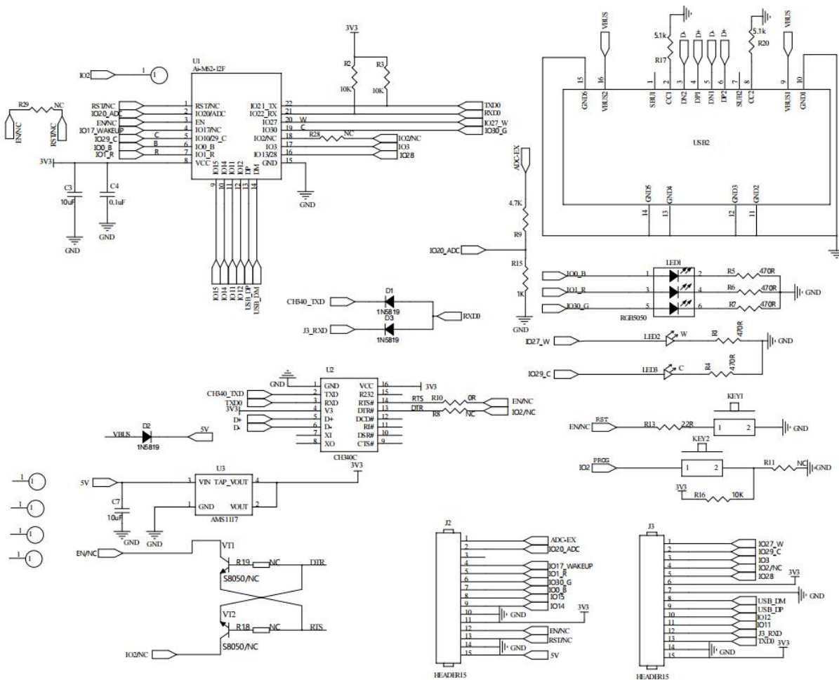
图 7 原理图
