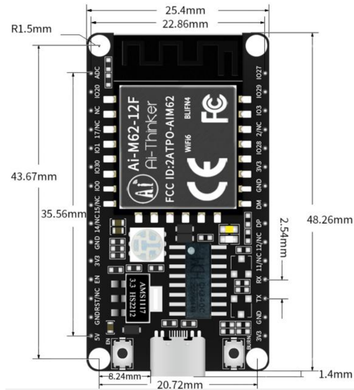
图 4 尺寸图
