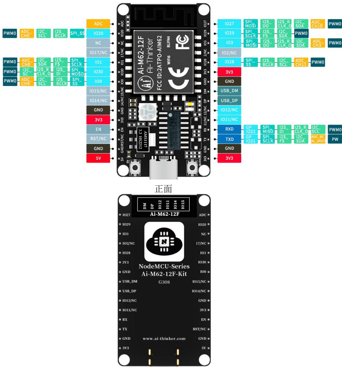
背面 图 6 管脚示意图
