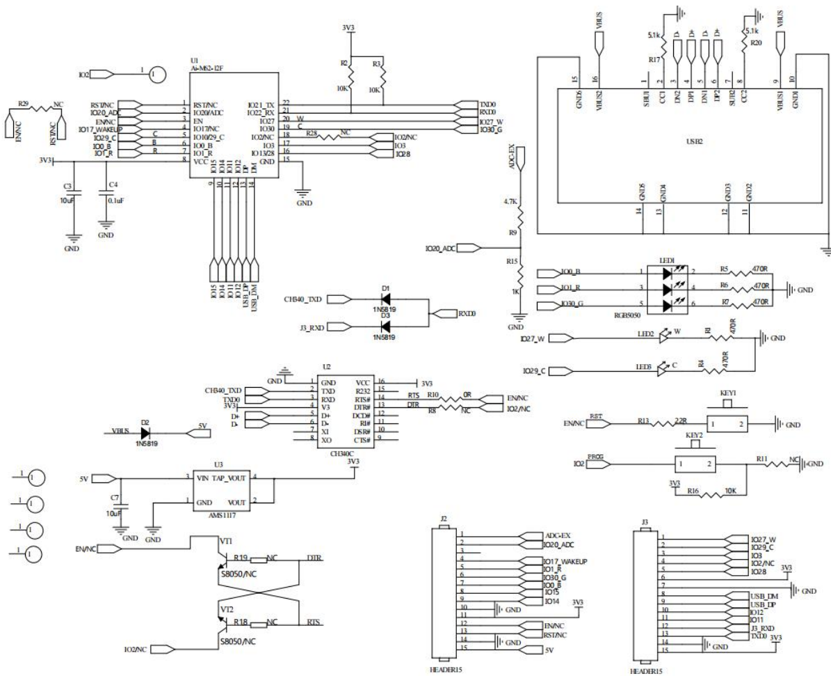
图 7 原理图
