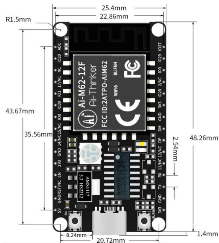
图 4 尺寸图
