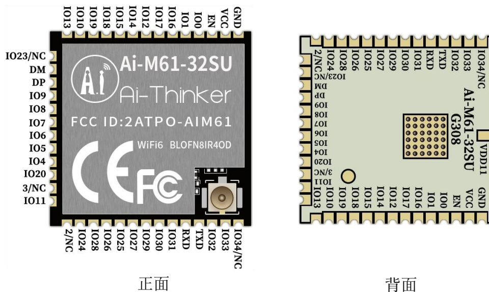
图 6 管脚示意图
