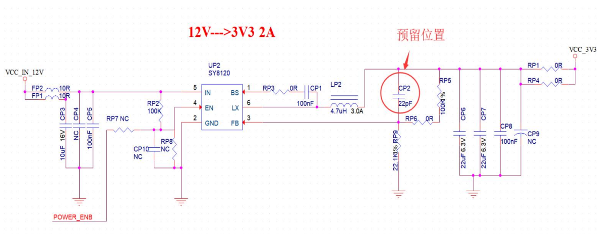
图 11 DC-DC 降压电路图
