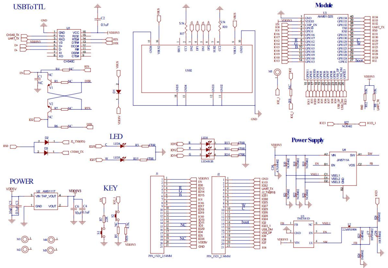
图 7 原理图
