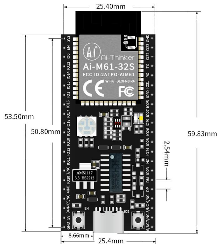
图 4 尺寸图
